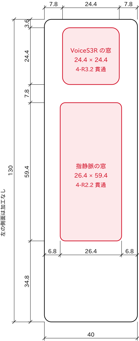
① カバー(外側=上から見た図)
