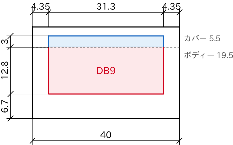
③ 端面(DB9 側)外から見た図
