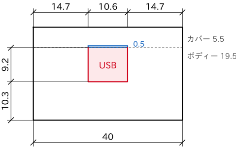
④ 端面(USB 側)外から見た図
