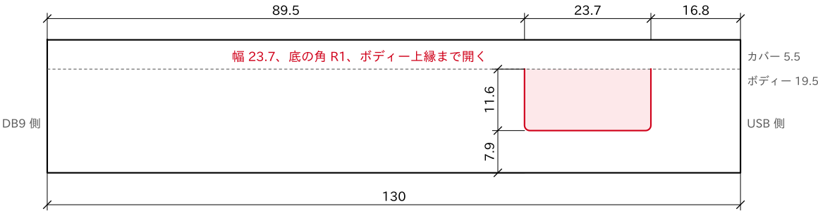
② 側面(①のカバーを上にして右側の面を外から見た図) — Grove コネクタとリセット用の切り欠き(1 つ)
